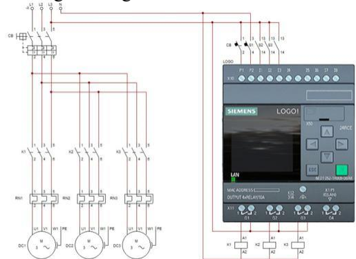
Hình 2.4. Sơ đồ mạch động lực điều khiển 3 động cơ thực hiện 2 chế độ
