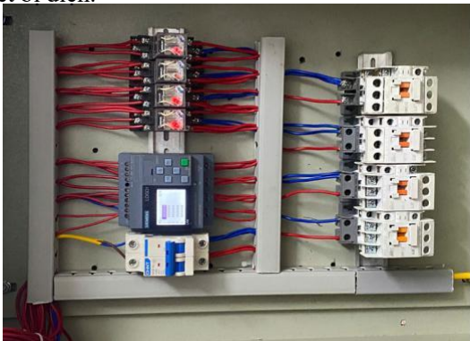
Hình 2.2. Mặt trong bộ thực hành PLC LOGO ! 230RCE SIEMENS
